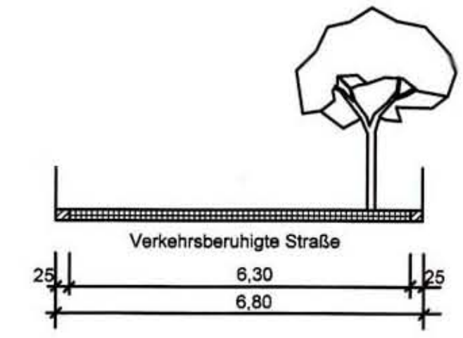
Schnitt B-B Straßen im Erschließungsgebiet ("Spielstraßen")
