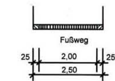
Allgemein: Schnitte der Fußwege
